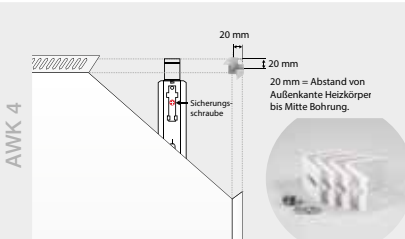
Winkel werden beidseitig (oberhalb vom Heizkörper) an der Wand befestigt.
