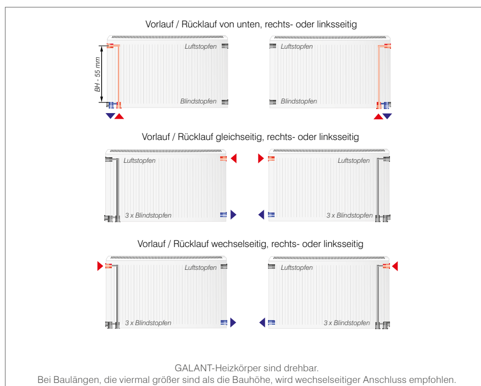
Typ 22 plus /Typ 22 Bautiefe 100 mm
