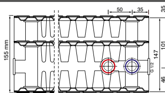
Typ 33 plus / Typ 33 Bautiefe 155 mm pr
