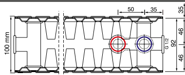
Typ 22 Bautiefe 100 mm
