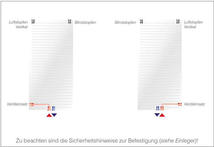
GALANT Vertikal Bautiefe 70 mm
