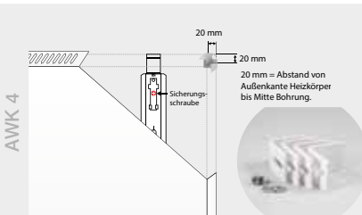
Winkel werden beidseitig (oberhalb vom Heizkörper) an der Wand befestigt.
