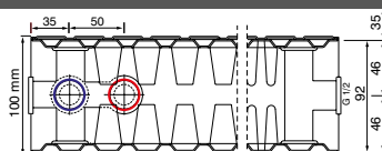
Typ 22 / Typ 22 plus Bautiefe 100 mm pl
