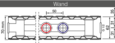
GALANT Vertikal Bautiefe 70 mm
