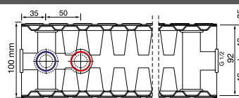
Typ 22 Bautiefe 100 mm pl
