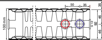
Typ 22 plus / Typ 22 Bautiefe 100 mm pr
