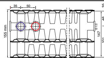
Typ 33 / Typ 33 plus Bautiefe 155 mm pl
