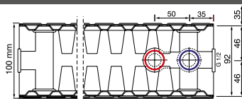
Typ 22 Bautiefe 100 mm pr
